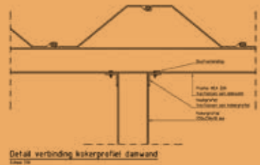
Detail verbinding kekerprofiel damwand L104 1/10
